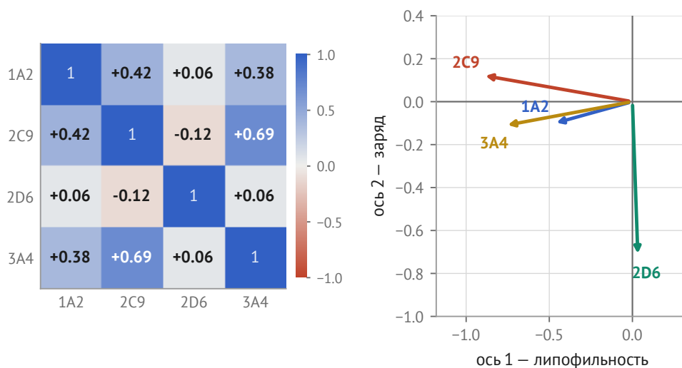
Рис. 7. Слева — ранговая корреляция \rho IC_{50} между ферментами, посчитанная по общим соединениям (от 230 пар у 2C9–2D6 до 473 у 2C9–3A4). Справа — нагрузки факторной модели ранга 2 на те же данные: каждая стрелка показывает, насколько фермент участвует в каждой из двух общих осей. Первая ось нагружает 2C9, 3A4 и слабее 1A2, на 2D6 стоит на нуле; вторая ось — почти исключительно 2D6.
